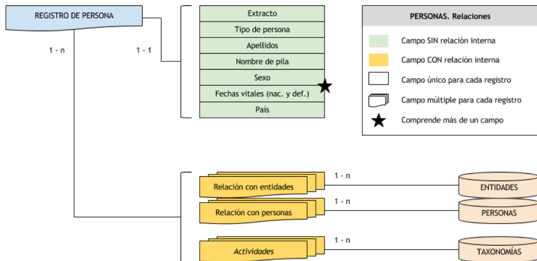
Fig. 3. Estructura de datos de la clase «Personas»
