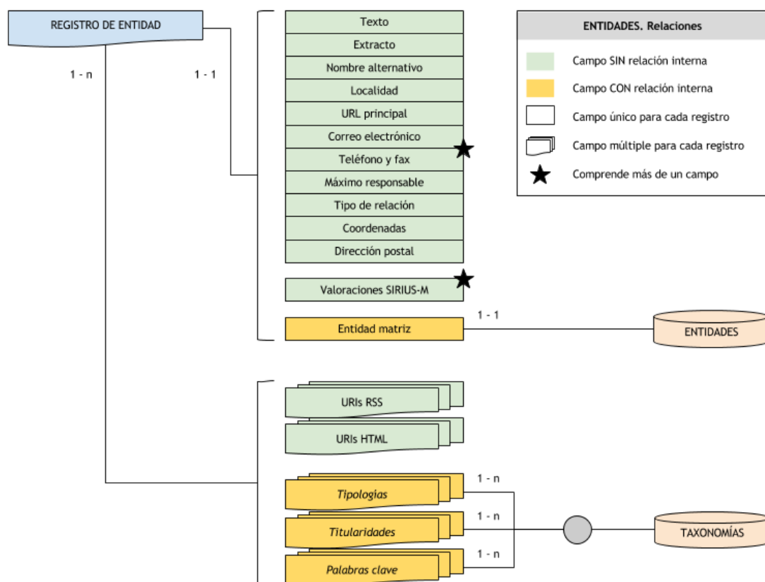
Fig. 2. Estructura de datos de la clase «Entidades»
